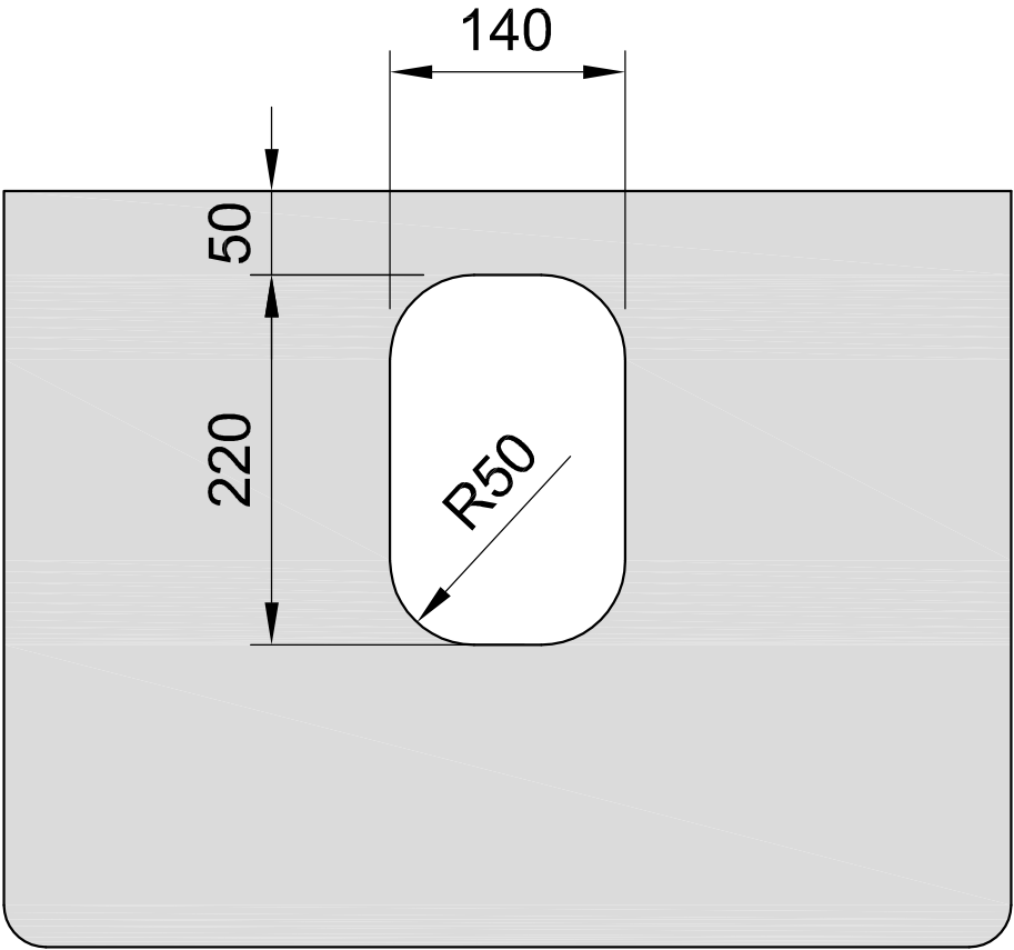
Detalle orificio encimera
